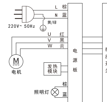
电气原理图
