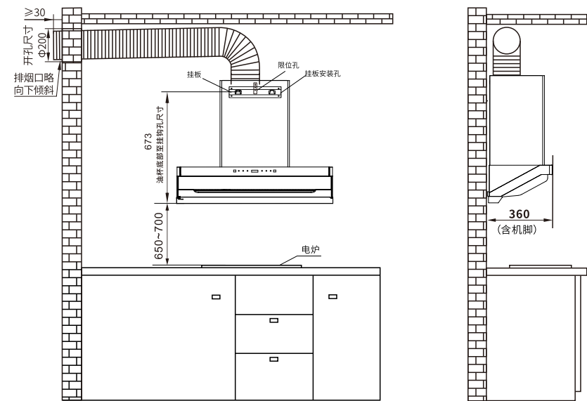
CXW-500-XK30-705A吸油烟机安装示意图
