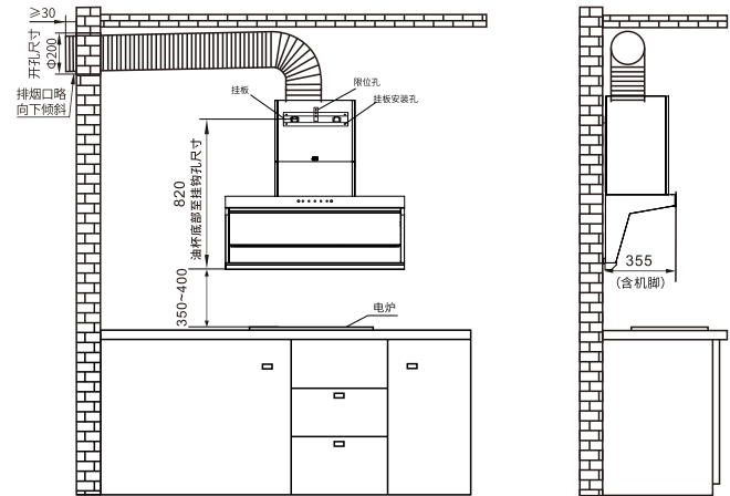
CXW-500-XL28-502吸油烟机安装示意图
