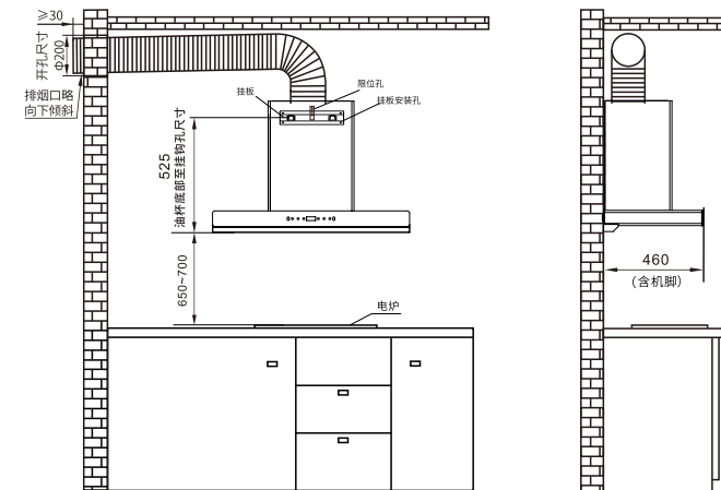
CXW-288-XT25-306吸油烟机安装示意图
